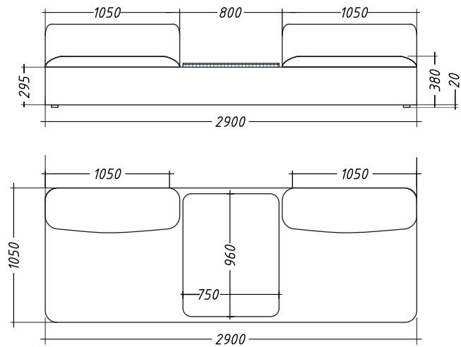
Вариант компоновки 3
